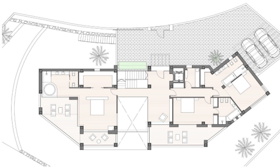
CASA GALERETES DISTRIBUCIÓN PLANTA PRIMERA (E:1/100)
