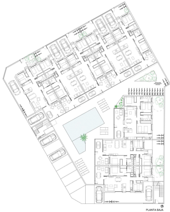
PLANTA BAJA
